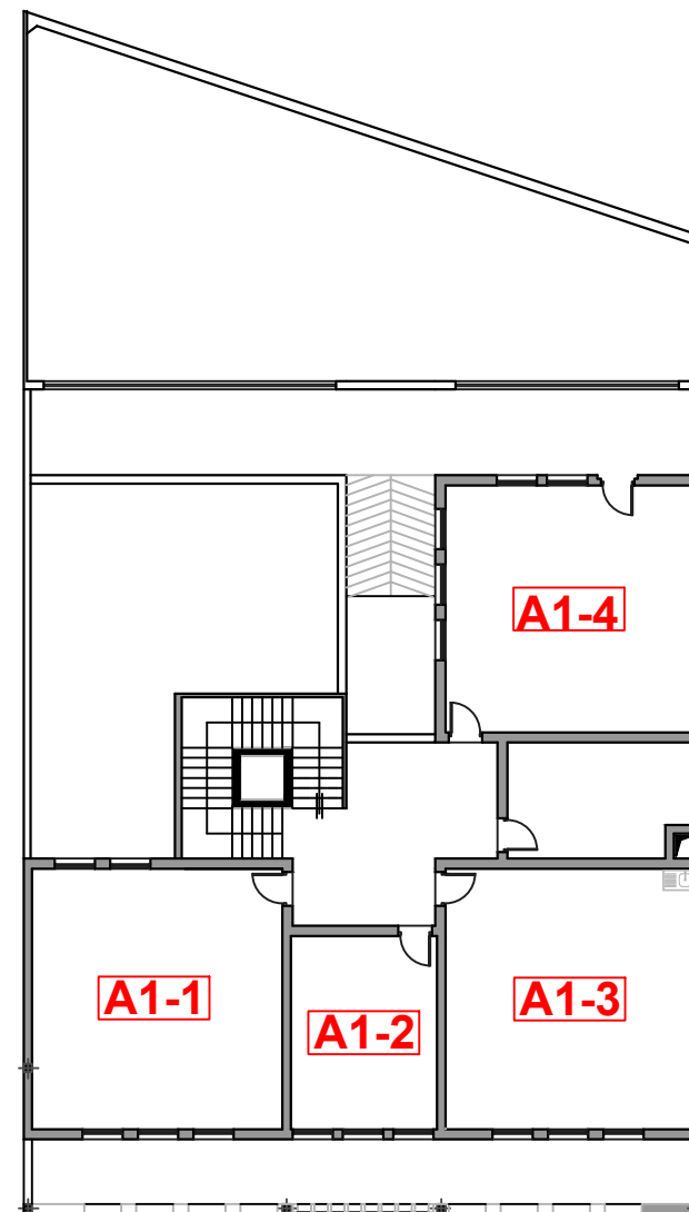
PLAN 1er ETAGE
